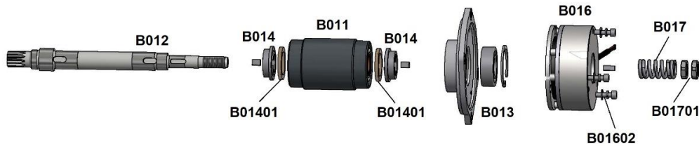
Einzelbremse
